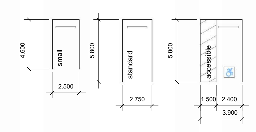
2 Vehicle Parking Stalls A103 / SCALE: N.T.S.
